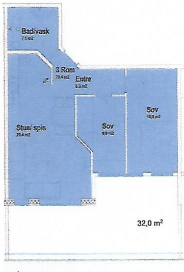
Leilighet M4 - 70,4 kvm.
