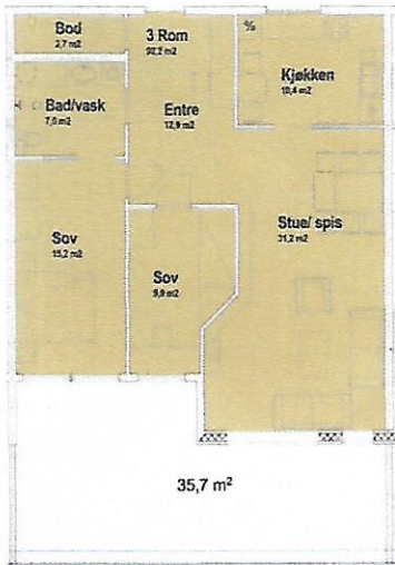
Leilighet L4 - 92,2 kvm.
